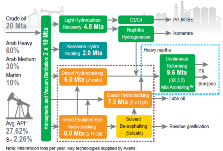
그림 02-11. Hengli PC의 중국 최초 COTC 설비
