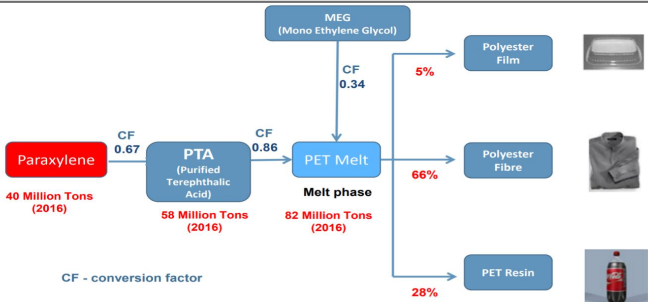
그림 02-2. PET Value Chain
